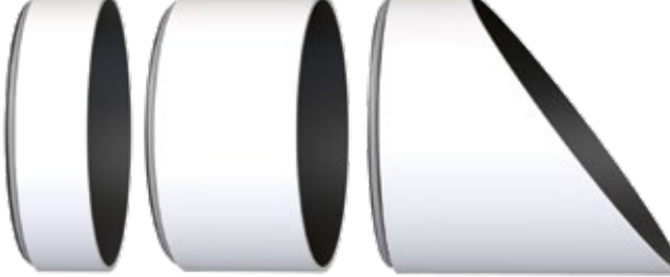
Abblending (Außenrohr pulverbeschichtet in Leuchtenfarbe, Innenseite oxidkeramisch beschichtet schwarz) Shutter (outer part powder-coated in spotlight colour, inner part oxide ceramic finish black)
